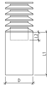
Säulenhut rund mit Standrohr aussen
