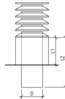
Lamellenhut rund mit Tablett (Flachdach 0°)
