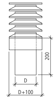
Lamellenhut rund mit Regenkragen und Steckmuffe
