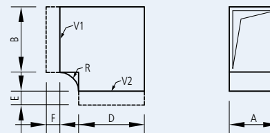
31 Übergangsknie (WA)
