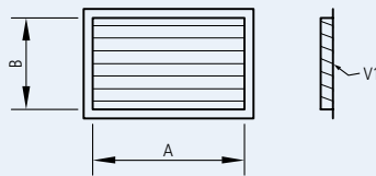
140 Wetterschutzgitter
