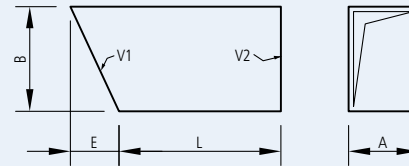
81 Hosenstück (HS)
