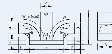
160 Abweiger
