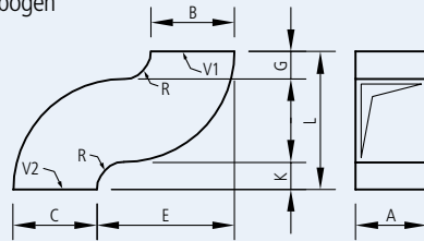
110 Doppelbogen
