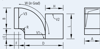
33 Abweiger rechts
