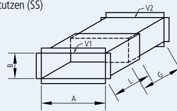
11 Schiebbestutzen (SS)
