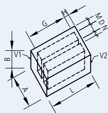
9 Schalldämpfer
