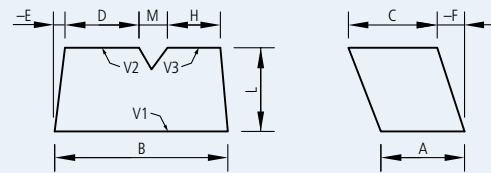
81 Hosenstück (HS)
