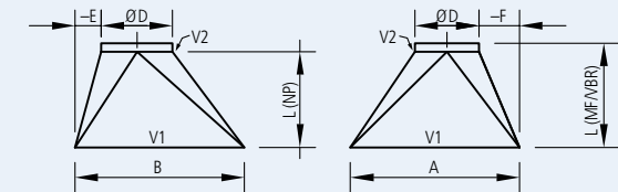
51 Übergang (RA)
