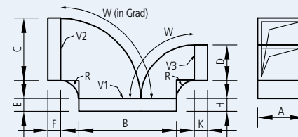
150 Abzweighbögen
