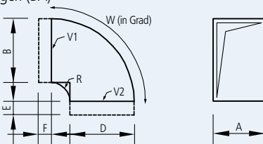
21 Übergangsbogen (BA)
