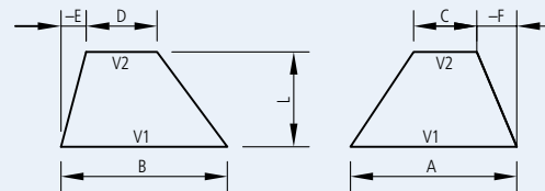
41 Konus (UA)
