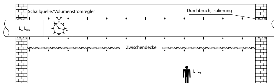
Bild 3: Darstellung Abstrahlgeräusch im Raum- Rohr nicht ummantelt
