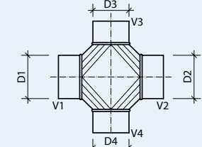
XCP/XCPU Kreuzstück 90°
