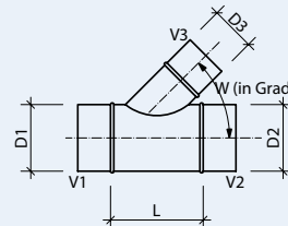
TV/TVU Abzweiger mit Winkel
