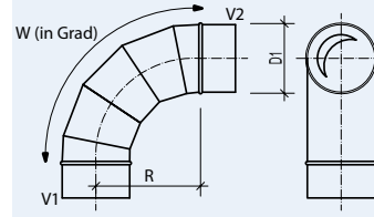
BF/BFU Segmentbogen
