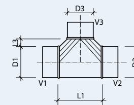
TC/TCU Abzweiger 90°
