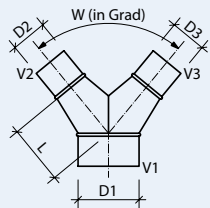
YV/YVU Hosenrohr
