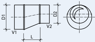
RL/RLU Reduktion exzentrisch
