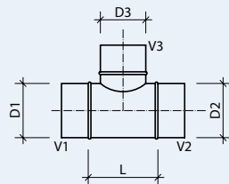
TCP/TCPU Abzweiger 90°
