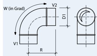
B/BU Bogen gepresst
